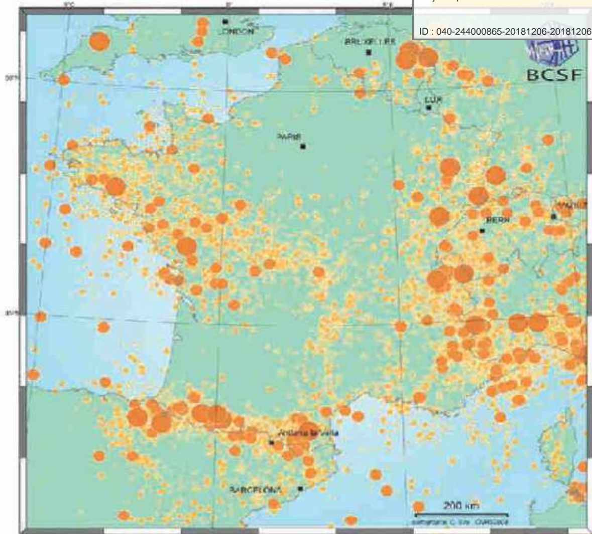
Epicentre des séismes selon leur magnitude ( M_L )
